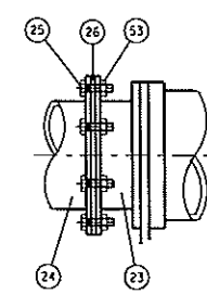
Detalj 4 1:5
