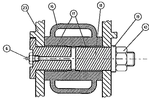
A - A 1:2
