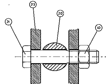
C - C 1:2
