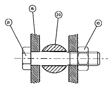
B - B 1:2
