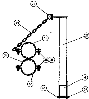
Detalj 5 1:5
